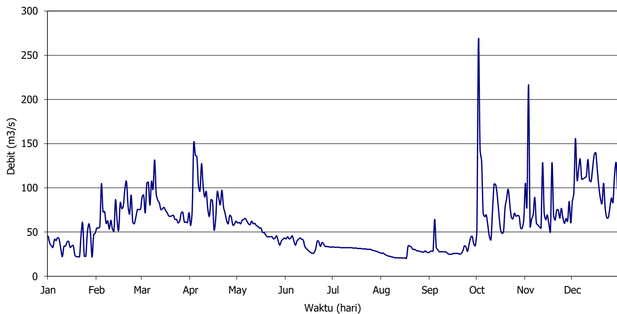
HIDROGRAF ALIRAN Cimuntur-Cibeka 2020
