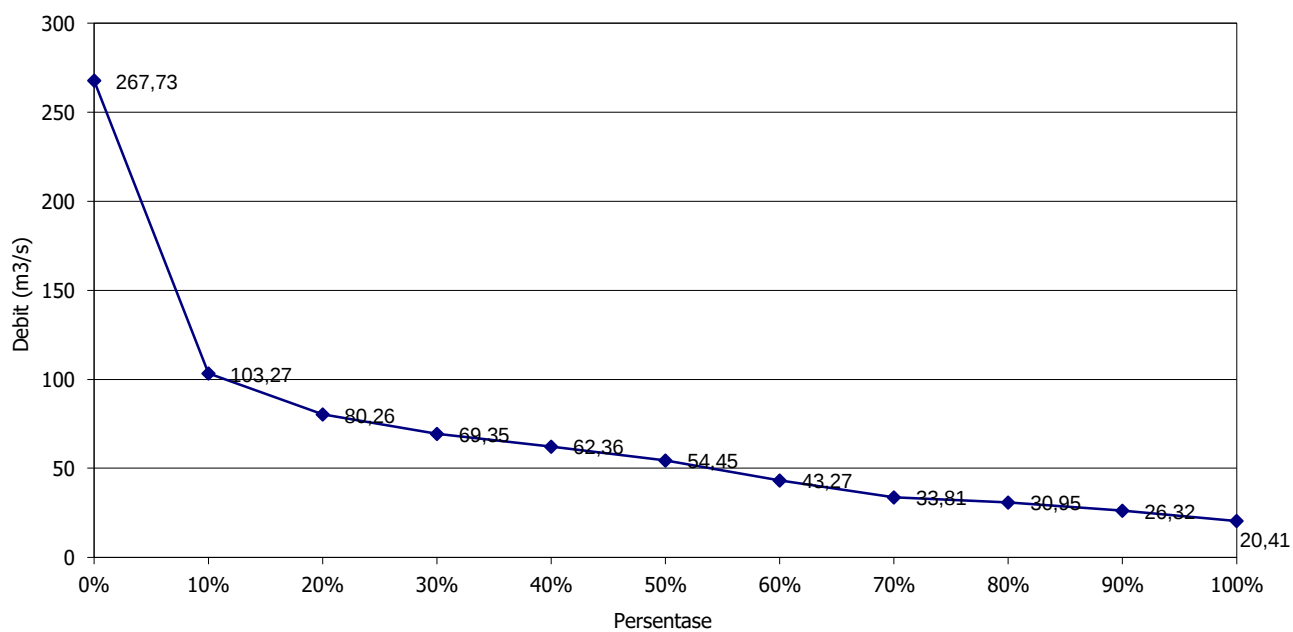
KURVA DURASI Cimuntur-Cibeka 2020
